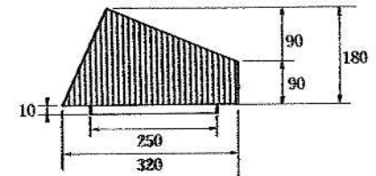
側面図
