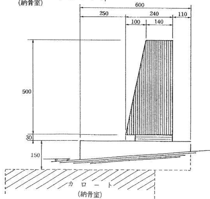
側面図
