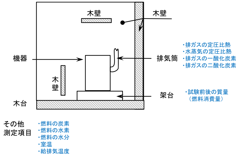
図 4-13 排気筒取付口が機器の側部にある場合の設置例
