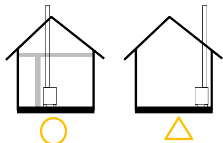
図 5-11 煙突の設置位置
