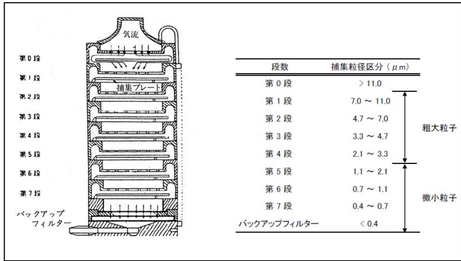
図 4-4 アンダーセンサンプラー断面図および格段の補修粒径区分
